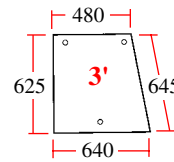
20/4043-2 (D7024, K303705) Lateral (izq.) Side (LH)
