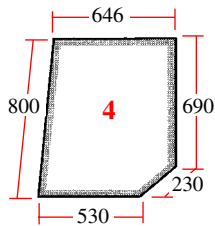
20/4035-1 (D7044, K965483) Puerta (superior izq.) Door (LH upper)
