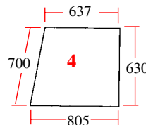
20/4028-2 (D7025, K303700) Puerta (dcha) Door (RH)
