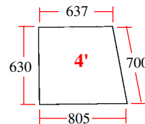
20/4039-6 (D7027, K303701) Puerta (izq.) Door (LH)
