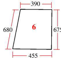
20/4041-5 (D7048/F) Lateral (fijo) (izq.o dcha) Side fixed (LH & RH)
