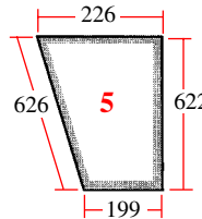
20/4037-1 (D7046, K965485) Puerta (inferior izq.) Door (LH lower)
