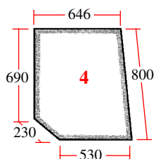
20/4034-1 (D7043, K965484) Puerta (superior dcha) Door (RH upper)
