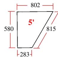
20/4029-2 (D7028, K303703) Puerta (izq.) Door (LH)
