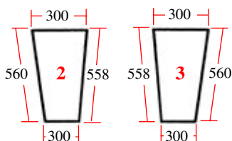
25/4012-29 (D7061, 1535088C1) Frontal inferior (drcha. y izq.) Front (RH & LH)
