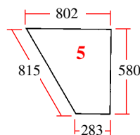
20/4038-6 (D7026, K303702) Puerta (dcha) Door (RH)
