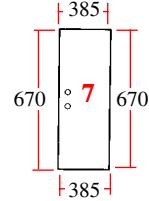
20/4040-3 (D7048/S) Lateral (deslizante) (izq.o dcha) Side sliding (LH & RH)
